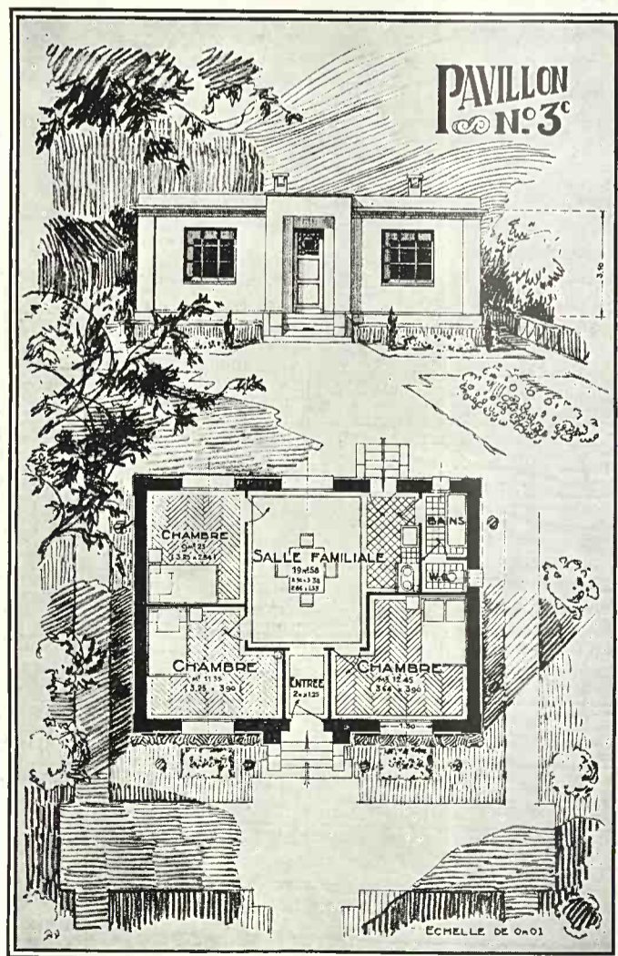
Relevé et plan d'un pavillon multicellulaire dit « type Loucheur n° 3 C ».
