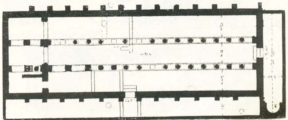
33. Planul basilicii din Tropaeum (CMI IV, 189).
