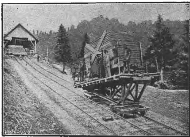
Transportul vagonului încărcat pe platforma funicularului.
