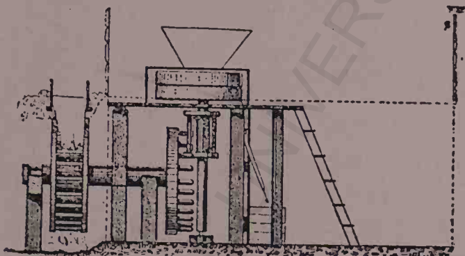
Fig. 75. Mecanica unei mori de apă din Nerej. (P. Stănculescu).
