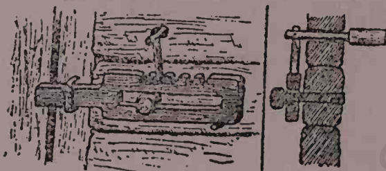
Fig. 73. Incuetoare de lemn (d. R. Vuia).
