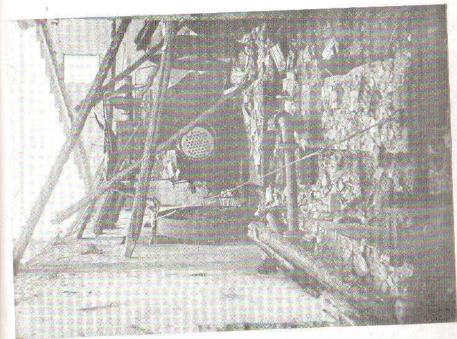
Mașinile moarei Victoria (Ismail) nimicite prin incendiu.
